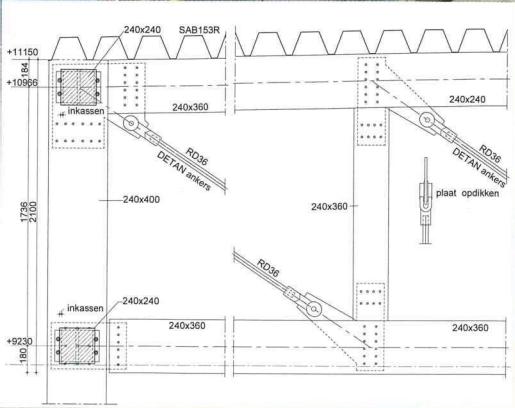
De knopen werden tot detail uitgeredend, de spanten werden met een 'zeeg' geconstrueerd.
