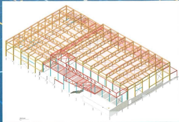
De vakwerken hebben enkele diagonalen of, op plekken met grotere windzuiging, gekruiste diagonalen.
